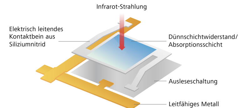
Schematische Darstellung eines Mikrobolometers.
