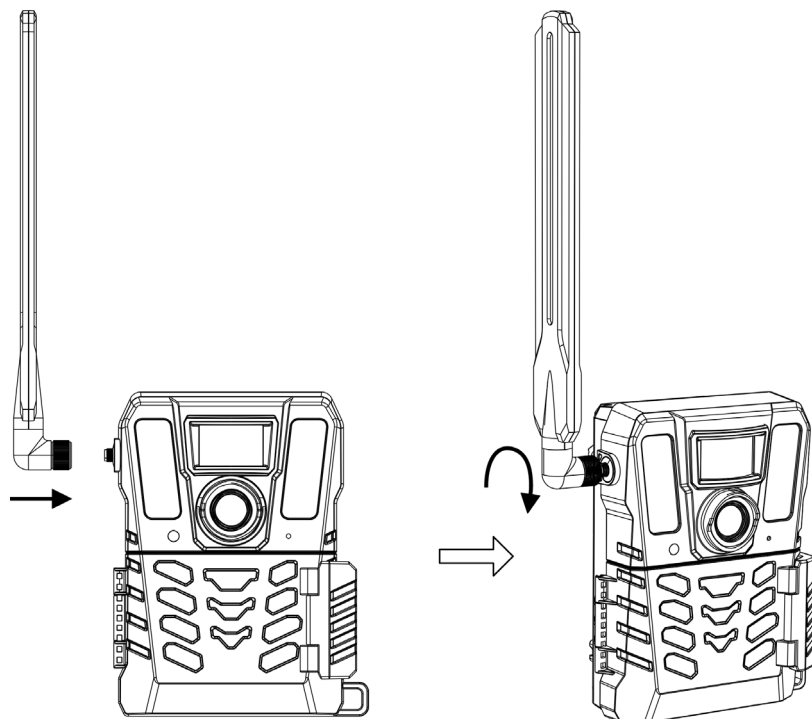
Abbildung 2-4 Antenne montieren
